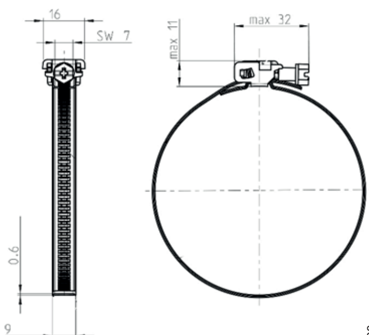
Måltegning
