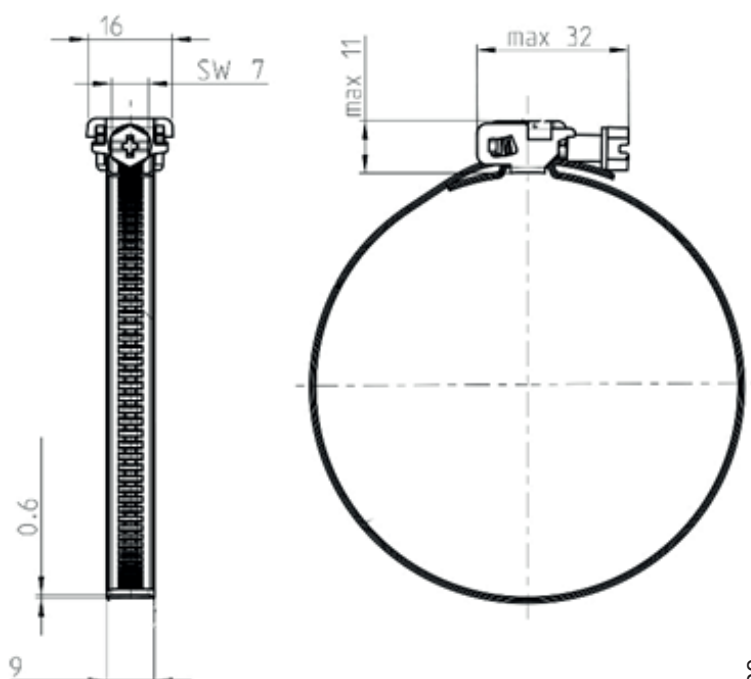
Måltegning
